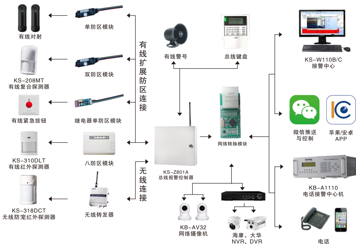
图一 系统工作示意图
