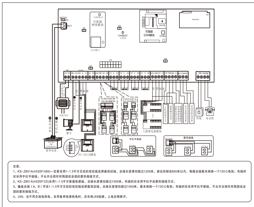
图二 主板接线图
